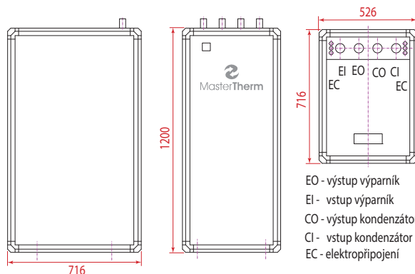
Rozměry a připojení modelů 22Z až 90Z:
