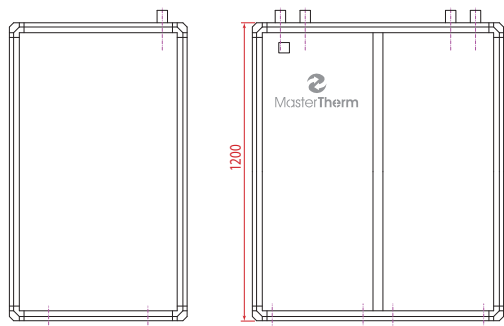
Rozměry a připojení modelů 120.2Z až 180.2Z:
